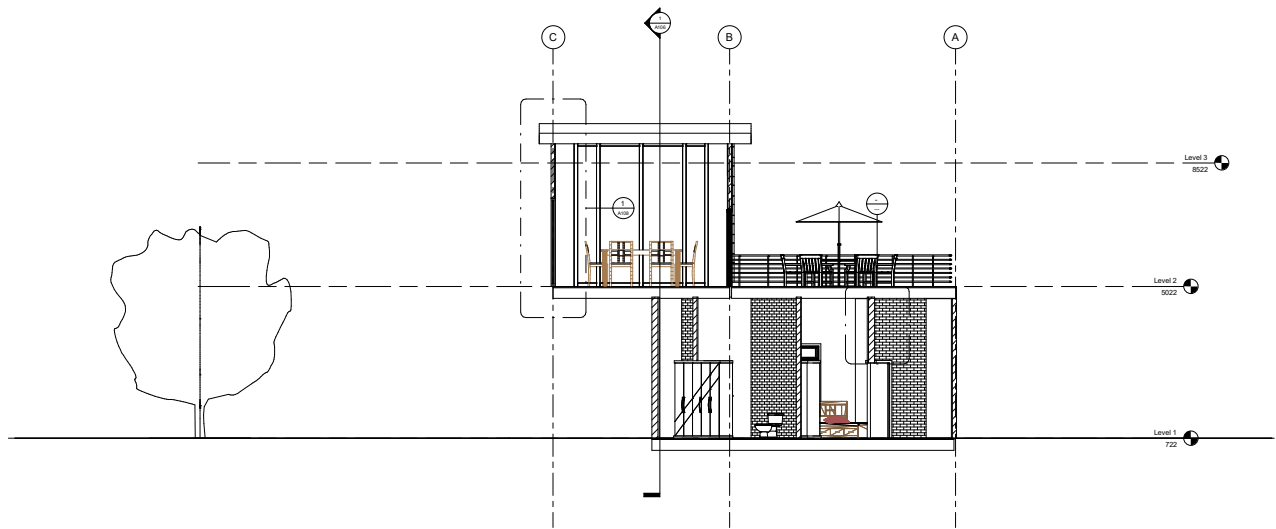
1 Section 1 1 : 50
