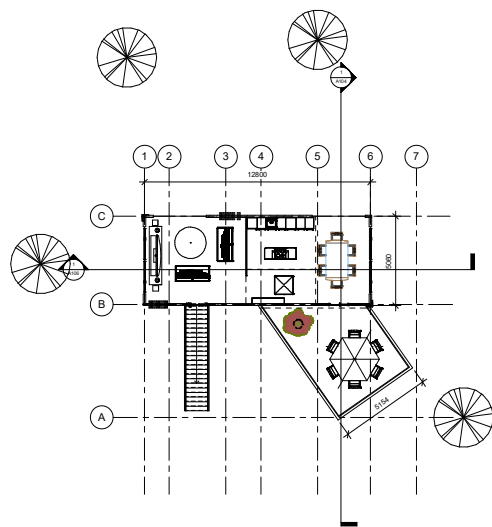
② Level 2 1 : 100
